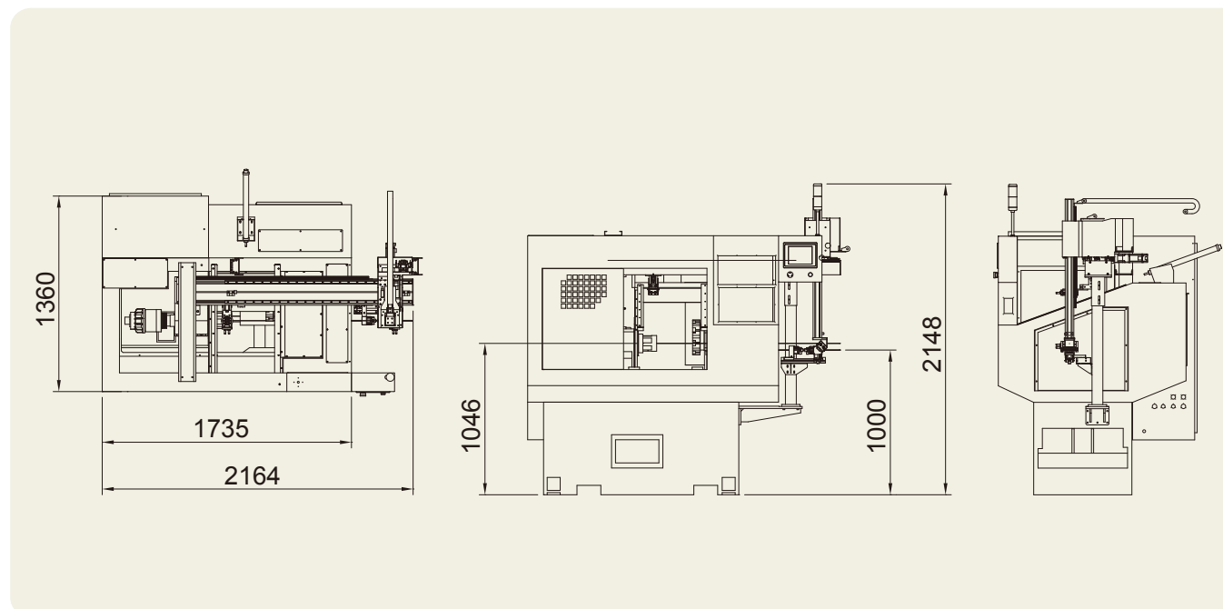
PLG-42 配門型機械手 PLG-42 With Gantry Robot
